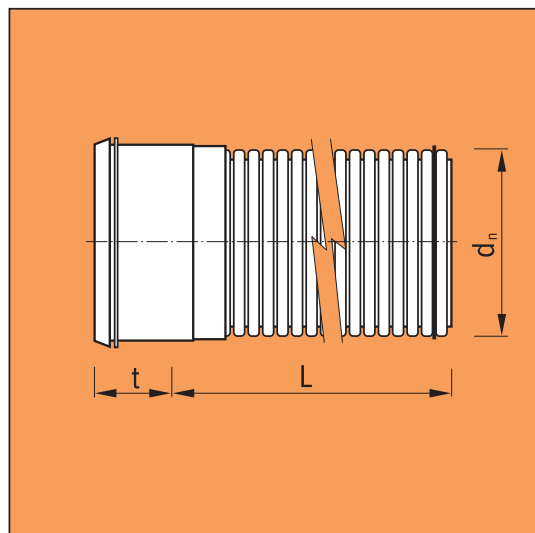
Прагма канализационная труба из ПП, двойные стенки
