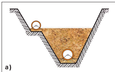
Ступенчатая траншея
