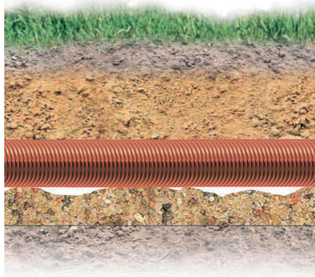
б) неправильно выполненное основание под трубой
